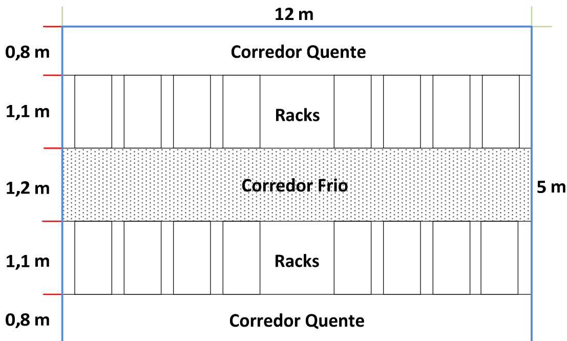
Figura 2 - Sugestão de leiaute 2
