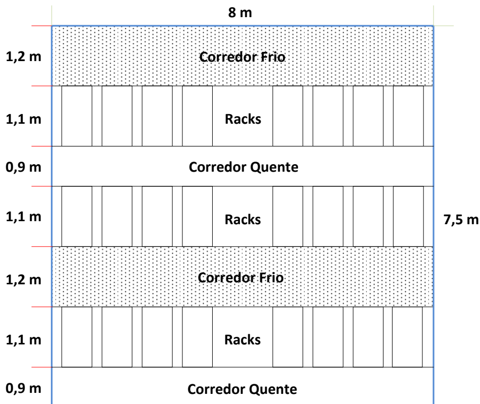
Figura 1 - Sugestão de leiaute 1
